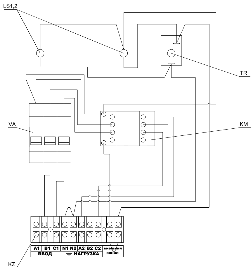
Рис.1 Схема монтажная ПУЭ-15
