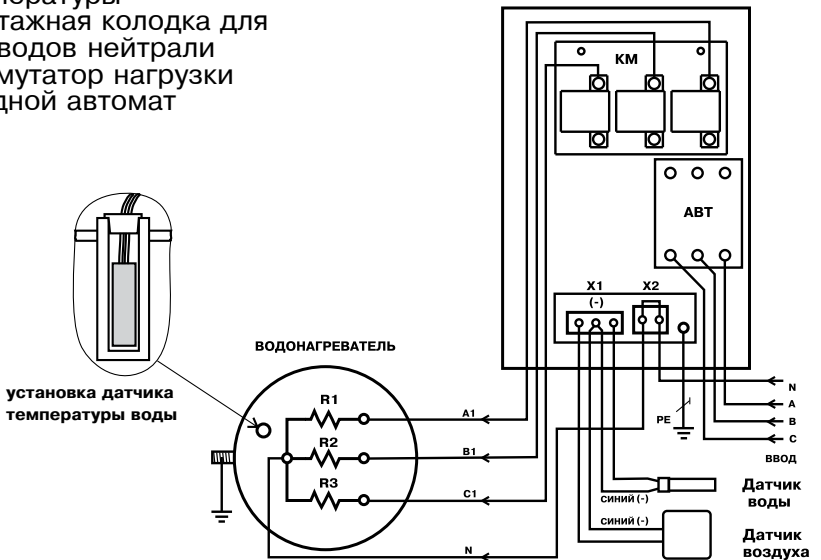
Рис.2 Схема подключения панели управления
